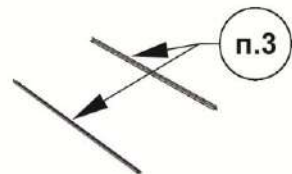
Рис.2 Расположить две стойки п.3 на поверхности для сборки.
