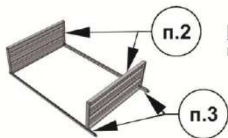
Рис.3 Наживить поочередно полки п.2 винтами М5х16 п.4 к стойкам п.3.
