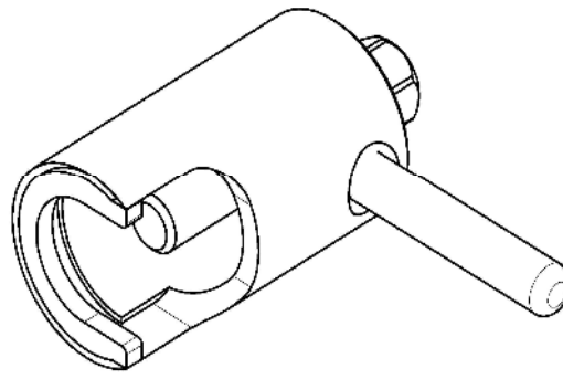
Рис. 18. Съемник крыльчатки.
